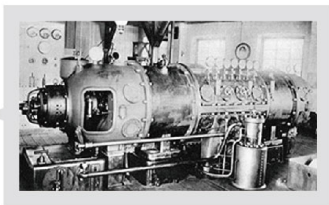
首台双螺旋涡轮机
