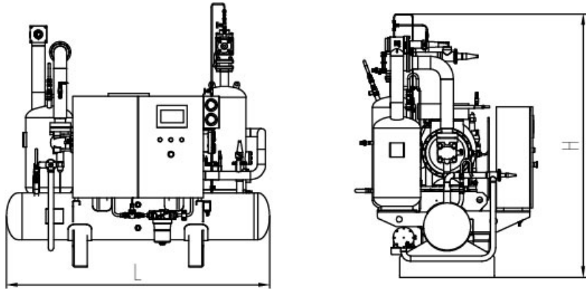
SW3H系列螺杆压缩机组外形图
