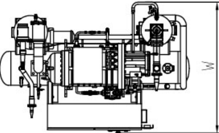
单机压缩机组
