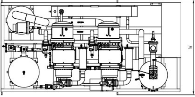
并联压缩机组
